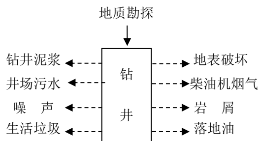
图 4-1 勘探井工艺流程及产污节点图
